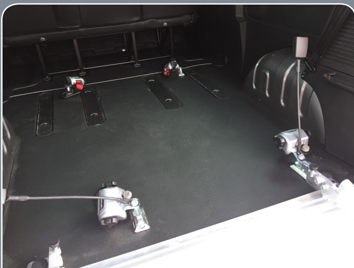
ENROULEURS DE FIXATION POUR LE FAUTEUIL ROULANT
